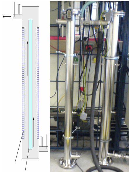
UV-Niederdruckstrahler Katalysator-Verbundmaterial
