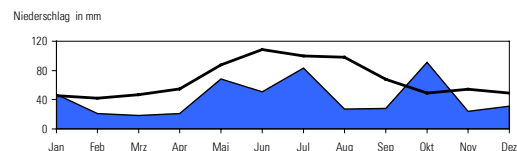
Abb. 4: Niederschlagsmengen 2003
