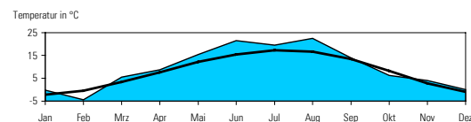
Abb. 3: Temperatur 2003
