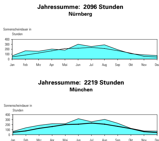
Abb. 2: Sonnenscheindauer 2003
